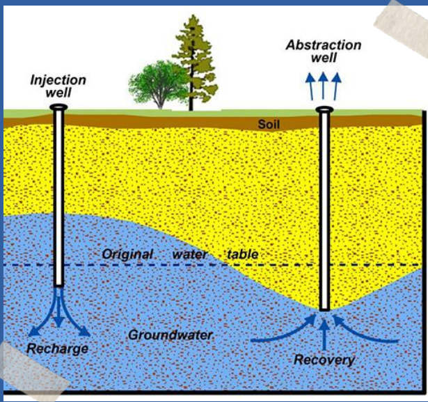
Schematische Darstellung der Grundwasseranreicherung mittels Brunnen in einem ungespannten Grundwasserleiter, modifiziert nach Managing Aquifers, 2023
