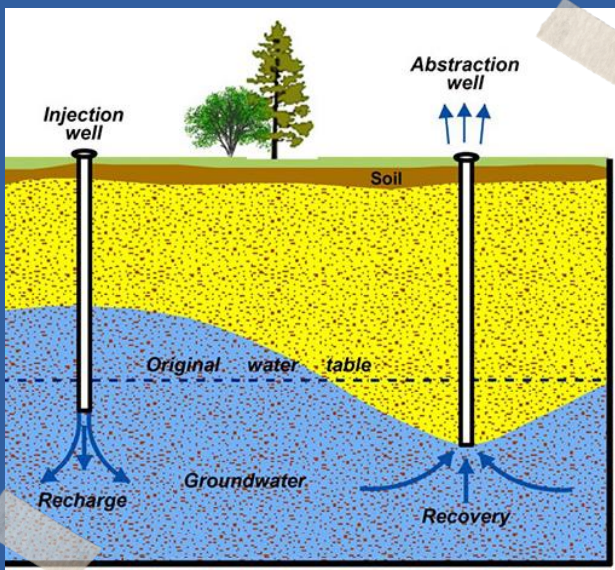
Schematische Darstellung der Grundwasseranreicherung mittels Brunnen in einem ungespannten Grundwasserleiter, modifiziert nach Managing Aquifers, 2023
