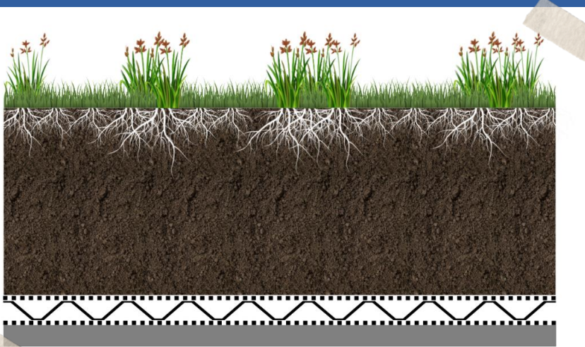
Intensives Gründach (© RPTU AMAREX)
