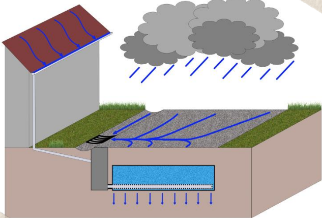
Versickerungsrigole + (© RPTU AMAREX)
