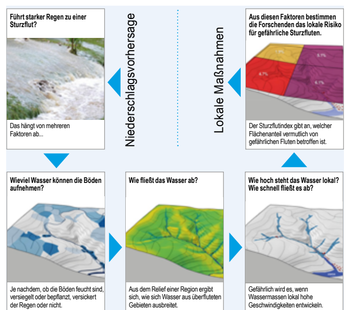
Abb.15 Schematischer Ablauf der Sturzflutvorhersage basierend auf dem SFI. (©AVOSS)
