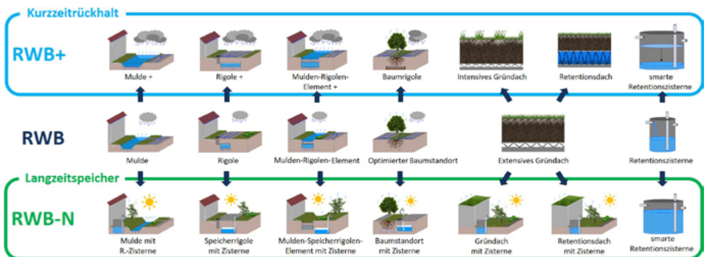
Abb.18 Funktionale Anpassung von Maßnahmen der Regenwasserbewirtschaftung (RWB) an die Wasserextreme Starkregen (RWB+) und Trockenheit (RWB-N) (©RPTU Kaiserslautern-Landau)
