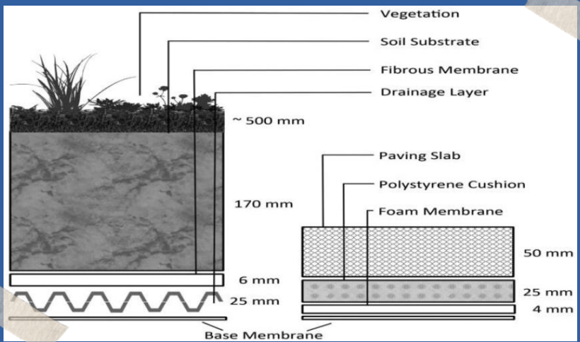
Querschnitt der Schichten des Gründachs (l.) und des konventionellen Dachs (r.) Bildquelle: Speak et al. 2013
